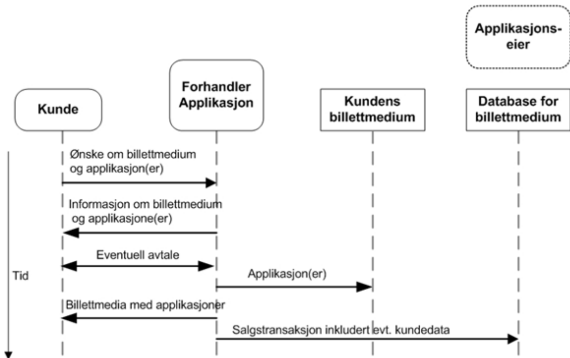
Figur 2-2 Anskaffelse av billettmedium med applikasjon på salgssted (terminal)
