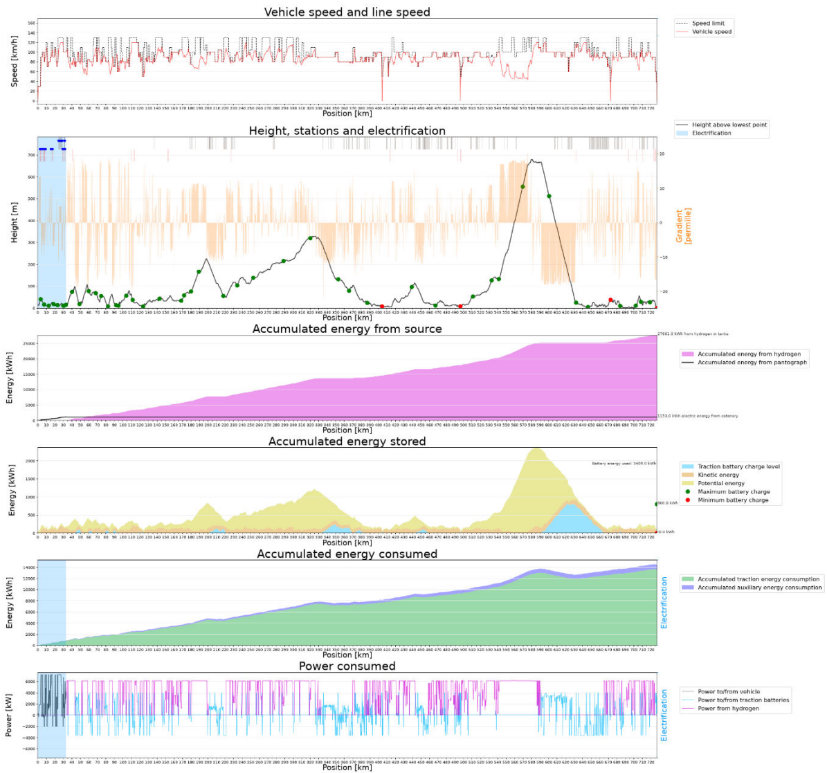
Figur 84: Simuleringsresultat for godstog GK25a, Trondheim – Bodø med konsept 2a, hydrogen. Grå ruter i graf nr 2 viser tunneler, og røde strek viser overgangsbruere. Blå prikk betyr at tunnelen eller overgangsbroen er på elektrifisert strekning.
