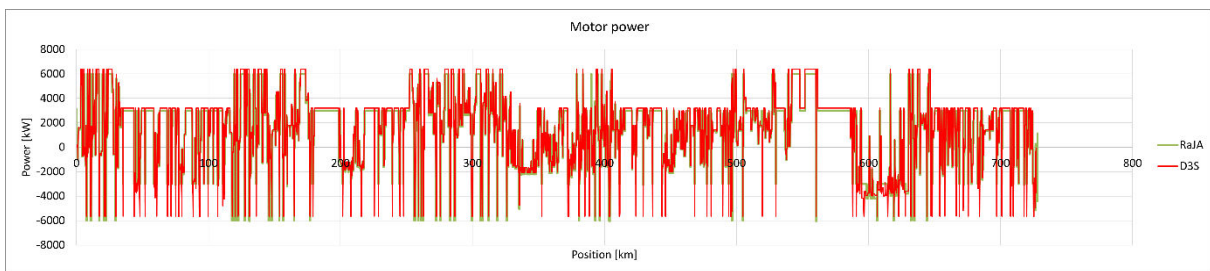
Figur 146: Sammenligning av simuleringsresultat. Godstog, nordgående, batteri (konsept 3). Effektforkbruk fra motorer.
