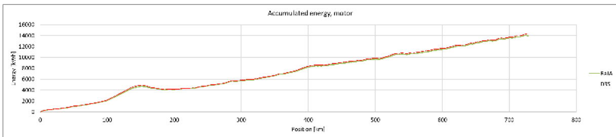
Figur 133: Sammenligning av simuleringsresultat. Godstog, sørgående, hydrogen (konsept 2a). Akkumulert energiforbruk fra motorer.
