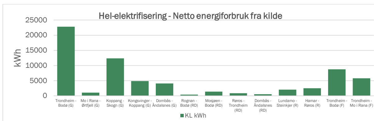
Figur 102 Konsept 4 - Elektrifisering. Netto energiforbruk ved kilde (kontaktledning). G=Godstog, RD=Regiontog i distrikt, R=Regiontog, F=Fjerntog.
