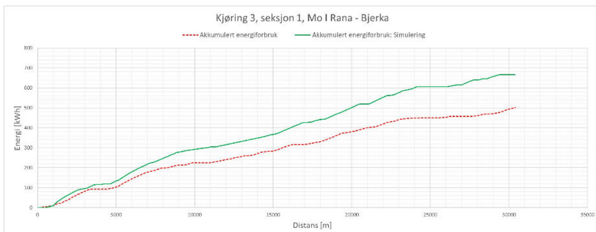
Figur 57: Validering - Kjøring 3, seksjon 1. Akkumulert energiforbruk.
