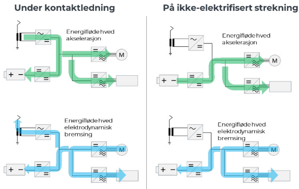
Figur 8: Illustrerer mulige energifloden ombord et batteri-kjøretøy.
