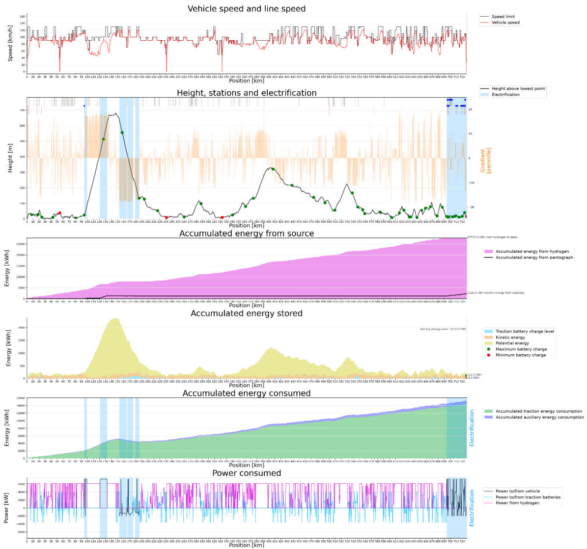
Figur 88: Simuleringsresultat for godstog GK25a, Bodø - Trondheim med konsept 2b, hydrogen med del-elektrifisering. Grå ruter i graf nr 2 viser tunneler, og røde strek viser overgangsbruere. Blå prikk betyr at tunnelen eller overgangsbroen er på elektrifisert strekning.
