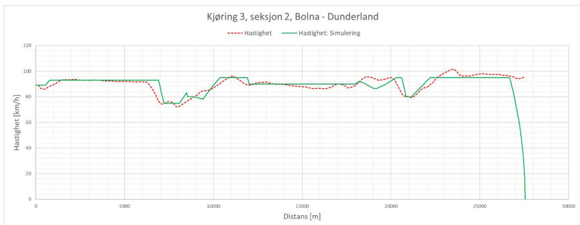
Figur 67: Validering - Kjøring 3, seksjon 2. Hastighet.
