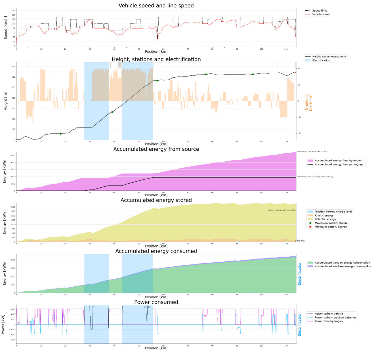
Figur 92: Simuleringsresultat for godstog GK23, Åndalsnes - Dombås med konsept 2b, hydrogen med del-elektrifisering. Grå ruter i graf nr 2 viser tunneler, og røde strek viser overgangsbruer. Blå prikk betyr at tunnelen eller overgangsbroen er på elektrifisert strekning.
