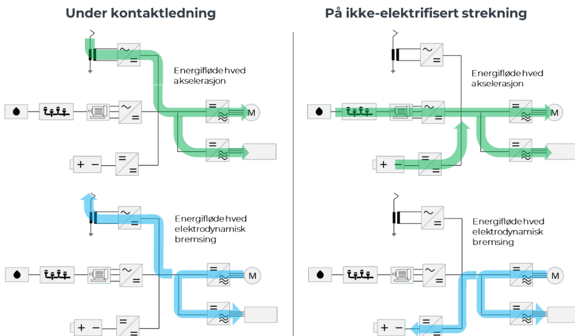
Figur 12: Illustrerer mulige energifløden ombord et diesel-kjøretøy.
