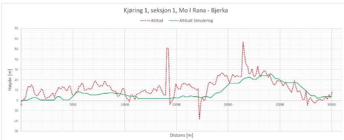
Figur 22: Validering - Kjøring 1, seksjon 1. Høydeprofil
