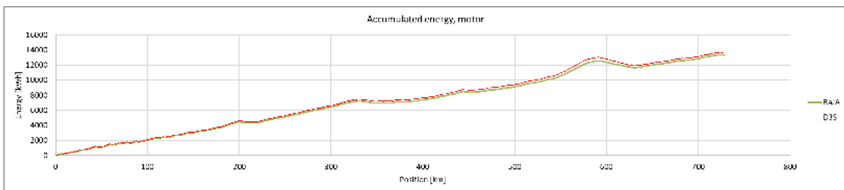
Figur 123: Sammenligning av simuleringsresultat. Godstog, nordgående, hydrogen (konsept 2a). Akkumulert energiforbruk fra motorer.
