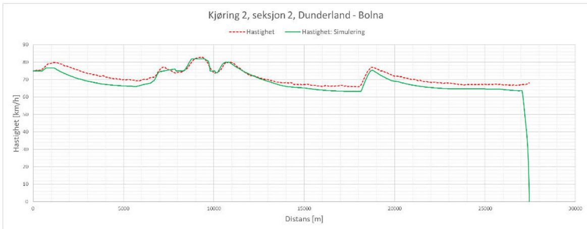
Figur 45: Validering - Kjøring 2, seksjon 2. Hastighet.
