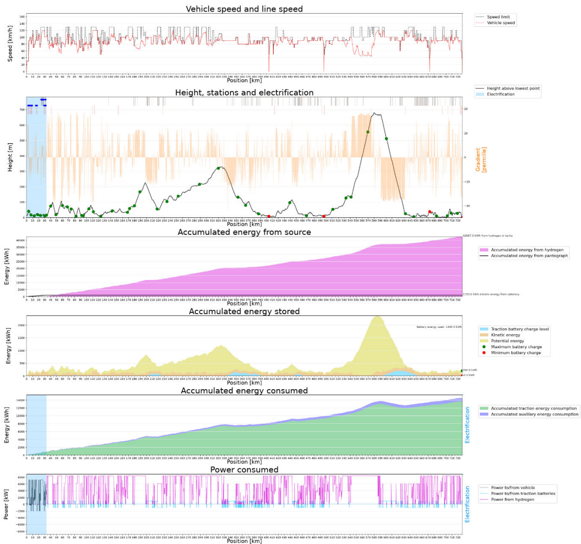
Figur 81: Simuleringsresultat for godstog GK25a, Trondheim – Bodø med konsept 0, diesel. Grå ruter i graf nr 2 viser tunneler, og røde strek viser overgangsbruer. Blå prikk betyr at tunnelen eller overgangsbroen er på elektrifisert strekning.
