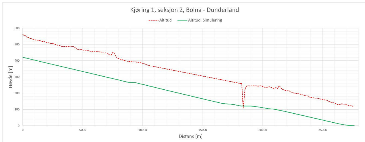
Figur 30: Validering - Kjøring 1, seksjon 2. Høydeprofil.
