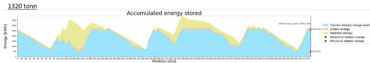
Figur 115: Batteri SoC for simulering med 1200 tonn (øvre) og 1320 tonn (nedre) for godstogslinje GK25a Bodø-Trondheim.
