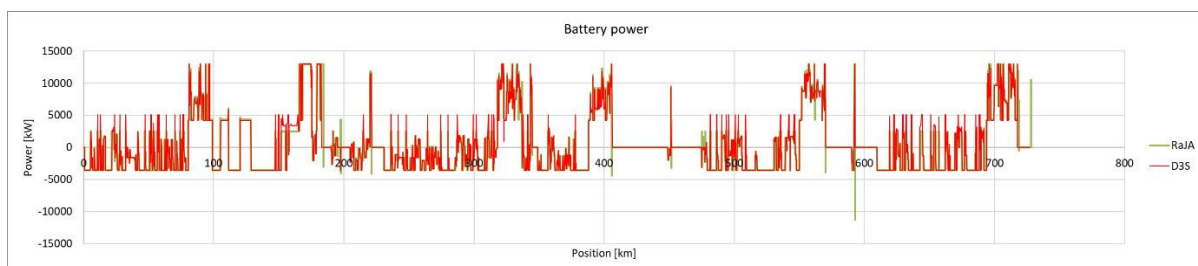
Figur 153: Sammenligning av simuleringsresultat. Godstog, sørgående, batteri (konsept 3). Batterieffekt.
