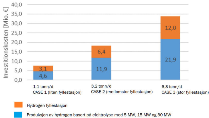
Figur 6: Investeringskostnader for fyllestasjonsinfrastruktur og elektrolyseenhet for forskjellige H 2 -produksjonskapasiteter i 2020. Referanse nr.4 side 21. (HYTRAIL)
