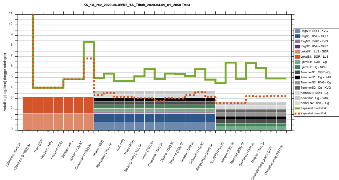
Figur 21 Togtilbud (søylor) og kapasitet (linjer) over hele døgnet i konsept K5.1. Rød stiptet linje viser kapasitet før tiltak og grønn linje kapasitet etter tiltak.
