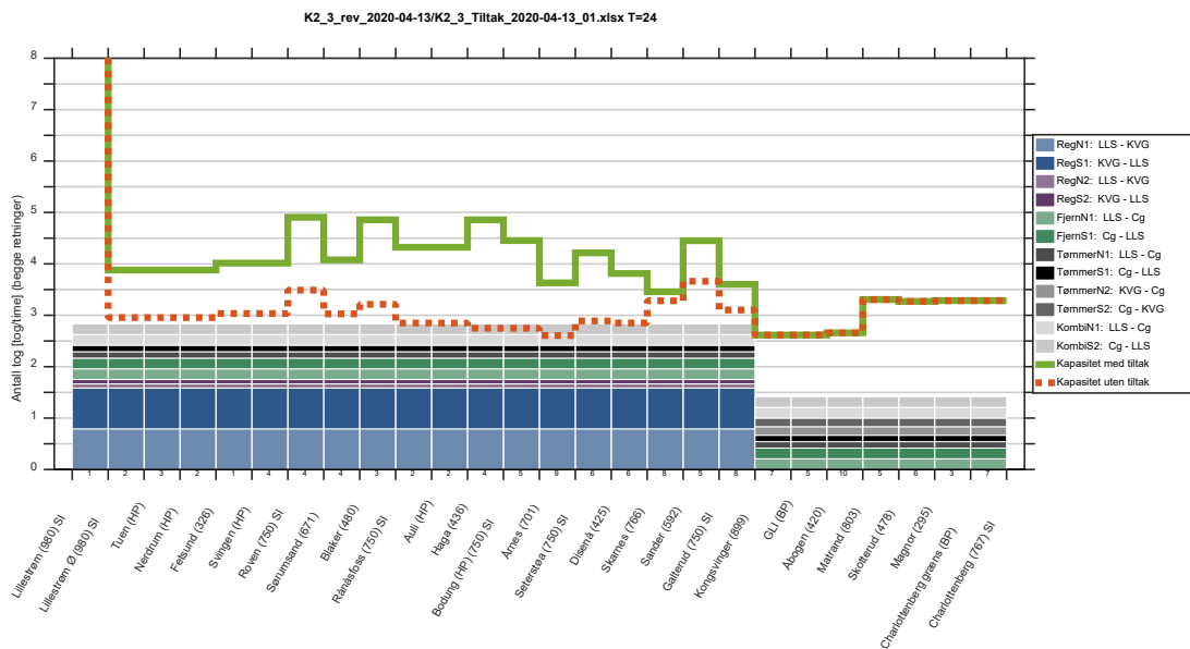
Figur 14 Togtilbud (søyler) og kapasitet (linjer) over hele døgnet i konsept K2.3. Rød stiptet linje viser kapasitet før tiltak og grønn linje kapasitet etter tiltak.
