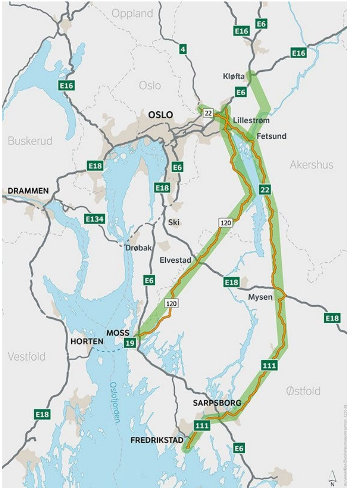
Figur 4-3. Prinsippkisse for KVU for vegforbindelse øst for Oslo, mellom E6 i Østfold og E6 på Romerike
