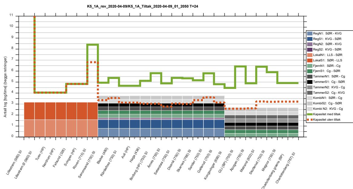
Figur 27: Togtilbud (søylor) og kapasitet (linjer) over hele døgnet i konsept K5.1. Rød stiplet linje viser kapasitet før tiltak og grønn linje kapasitet etter tiltak. Oversikt over rushperioden finnes i underlagsrapporten med kapasitetsberegninger.
