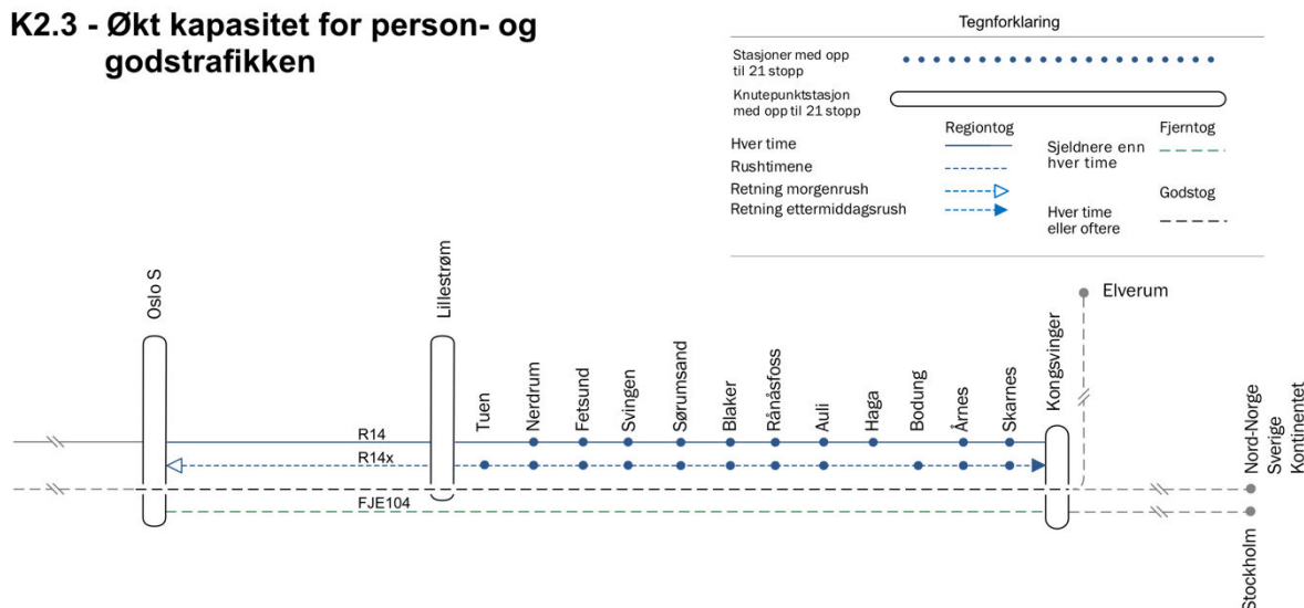
Figur 18: Prinsippskisse for konsept 2.3 Økt ombordkapasitet for både person- og godstog med dagens stoppmønster.
