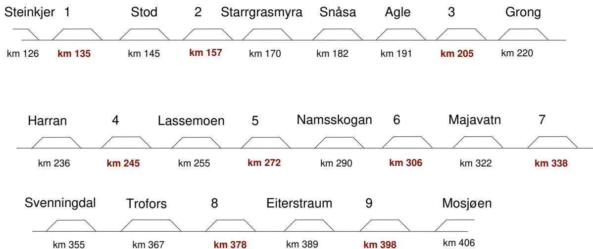
Figur 3-5: Skematisk fremstilling av Nordlandsbanen fra Steinkjer til Mosjøen. Rød skrift angir nytt kryssingsspor.
