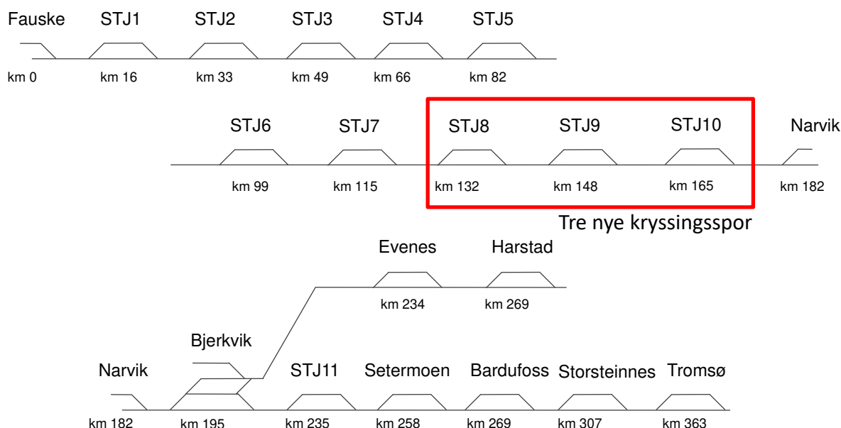
Figur 3-4: Skjematisk fremstilling av strekningen Fauske til Tromsø og Harstad. I rød ramme vises de 3 nye kryssingssporene som anbefales tilført strekningen for å gjøre rutemodellen robust.
