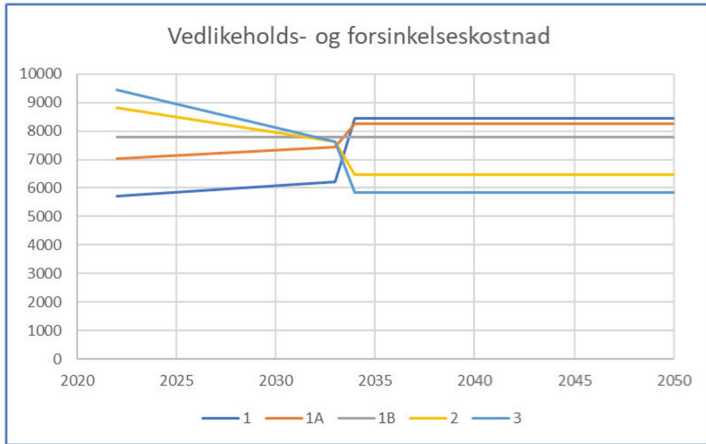
Figur 8 Framskriving av årlige samlede vedlikeholds- og punktlighetskostnader.
