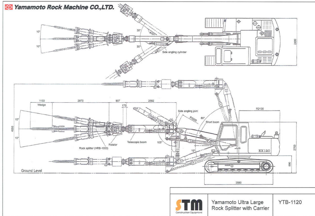
Figur 22: Figuren viser en gravemaskin utstyrt med en hydraulisk bergbryter av kilettype
