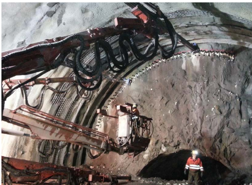
Figur 6: Etablering av rørspiling ved passering av svakhetssone i Holmestrandtunnelen
