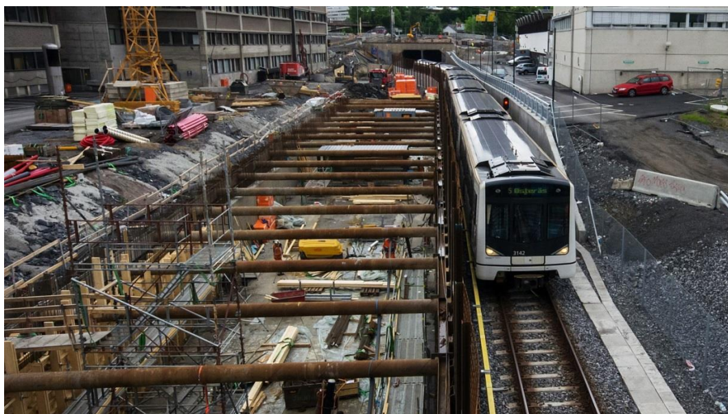
Figur 3: Byggegrøp med innvendig avstivet spunt for løsmassetunnel på Lørenbanen. Foto: Geovita
