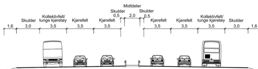
Figur 14: Typisk snitt for utvidelse fra 4- til 6-felts vei.
