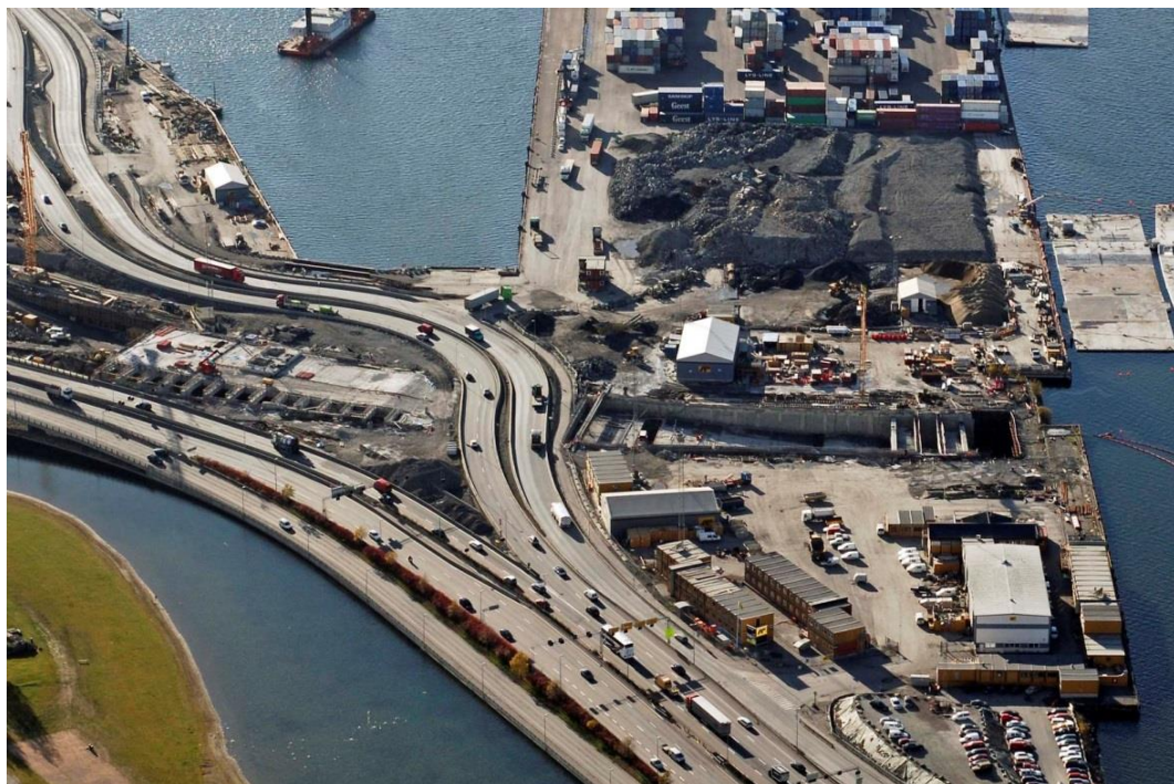
Figur 2: Byggegrøp for løsmassetunnel med slissevegger ved Sørenga. Foto: Statens vegvesen
