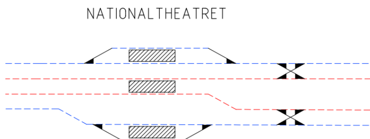
Figur 55: Skjematisk plan for Nationaltheatret stasjon med 6 spor til plattform
