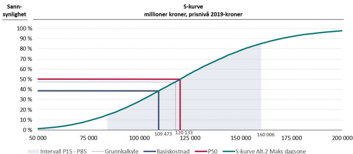
Figur 6 - S-kurve Alternativ 2.
