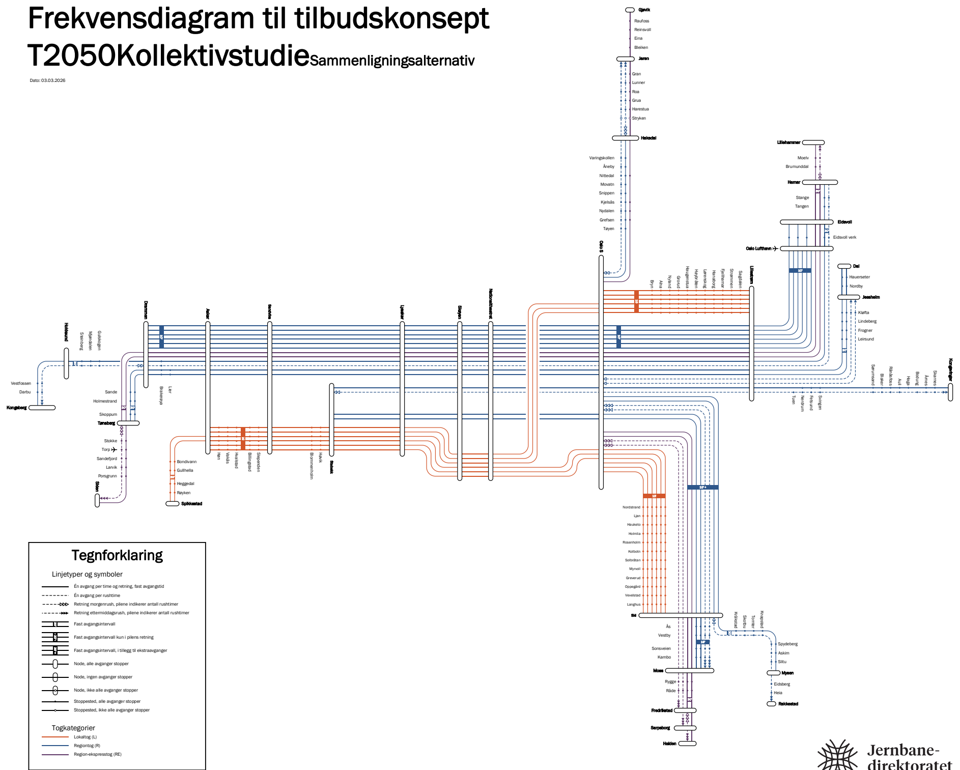
Figur 1: Frekvensdiagram Sammenligningsalternativ
