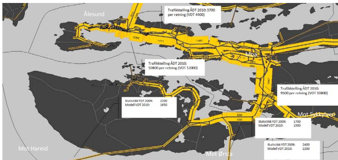
Figur 3-5 Tellinger og modellberegninger for nettverket i Ålesund og omegnskommuner. Døgntall 2010.
