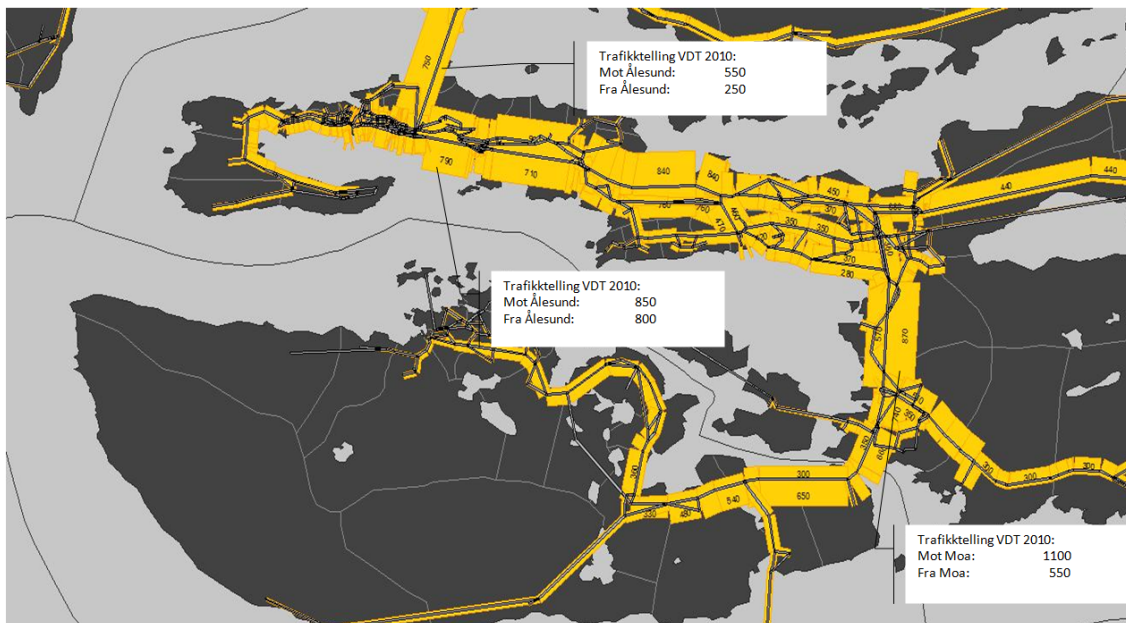
Figur 3-6 Telling og modellberegninger for nettverket i Ålesund og omegnskommuner. Maksimaltrafikktime morgenrush 2010.
